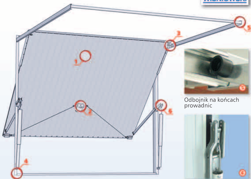
Łatwy sposób regulacji naciągu sprężyn
